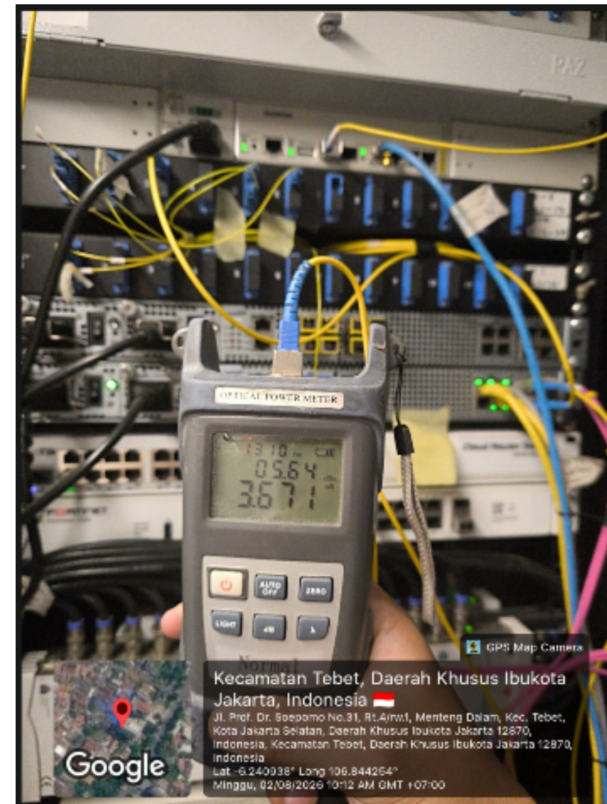
Redaman keluaran dari sfp olt dasan
